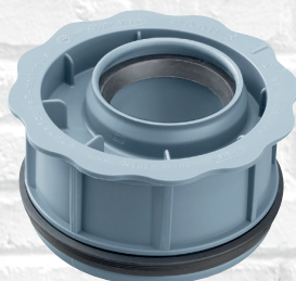
Articolo n. 6680 - DN 110/50
