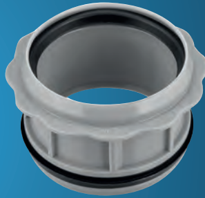
Art.-Nr. 6672 OHA-RDST- Innenreduzierung DN 110 / DN 90
