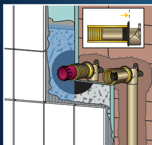
b: pro běžnou vyžděnou stavbu
