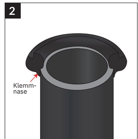
2. Ring mit Nase auf Spitzende klemmen.
